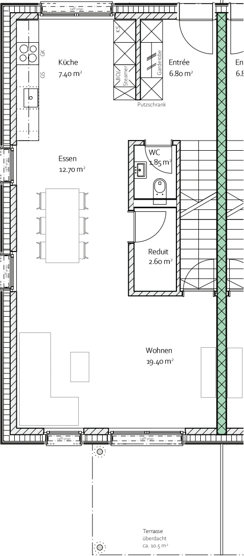
Erdgeschoss
